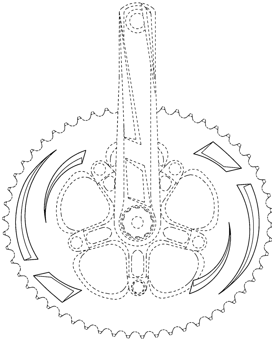
仰視圖
